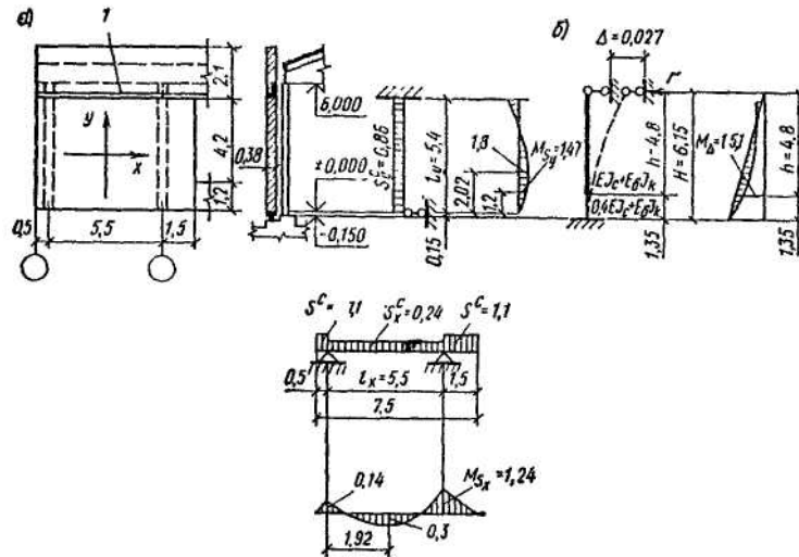
a - от действия местной сейсмической нагрузки; б - от перемещения стены вместе с каркасом; в - антисейсмический пояс
