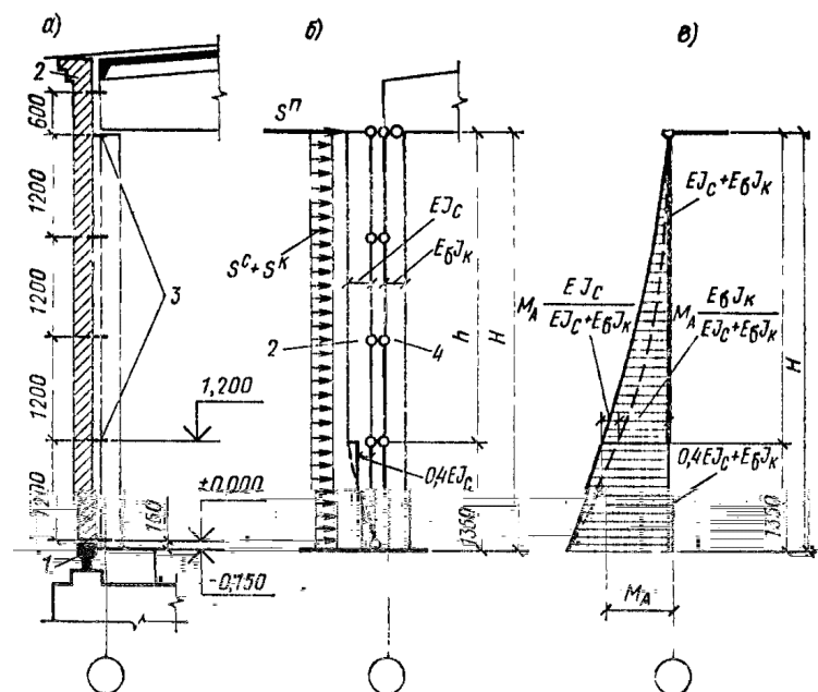
а - поперечный разрез; б - расчетная схема; в - эпюра изгибающих моментов; - фундаментная балка; - самонесущая кирпичная стена; - анкеры крепления стен; - колонна
