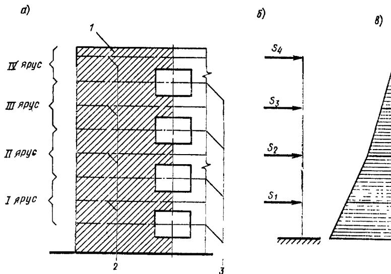
а - элемент фасада стены; б - расчетная схема; в - эпюра M ; - оси проемов; - оси горизонтальных поясов; - простенки
