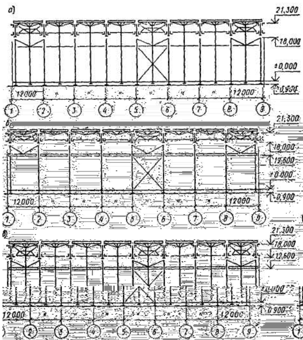
a - по оси А; б - по осям В и В; в - по оси Г
