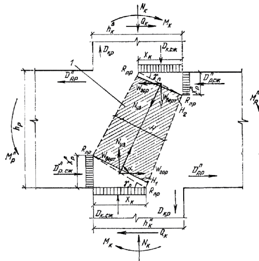
- расчетная призма
