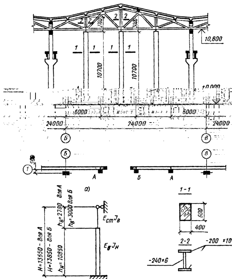
а - расчетная схема фахверковой колонны
