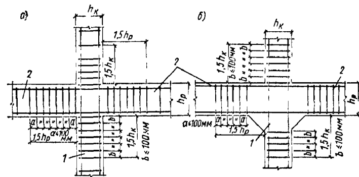
a - при бесконсольном сопряжении; б - при опирании ригелей на короткие консоли колонны; - колонна; - ригель
