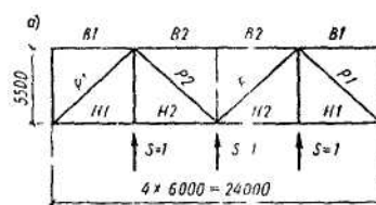
а - геометрическая схема связи; б - схемы расположения сейсмических нагрузок; в - усилия в связевой ферме от единичных нагрузок
