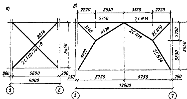
а - по оси А и Г; б - по оси В и В; - стальные связи
