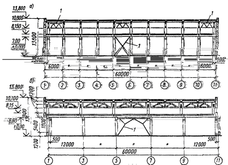
а - по оси А и Г; б - по оси В и В; - стальные связи
