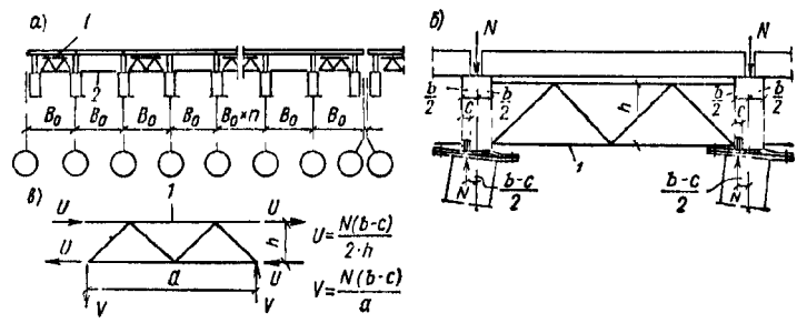
a - схема покрытия; б - схема деформированного элемента покрытия; в - расчетная схема связи; - вертикальная связь; - распорка
