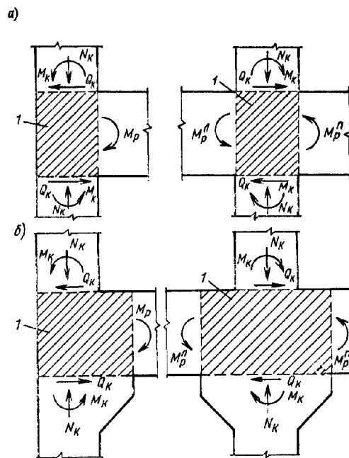
a - при бесконсольном сопряжении; б - при опирании ригелей на короткие консоли колонны; - колонна; - ригель
