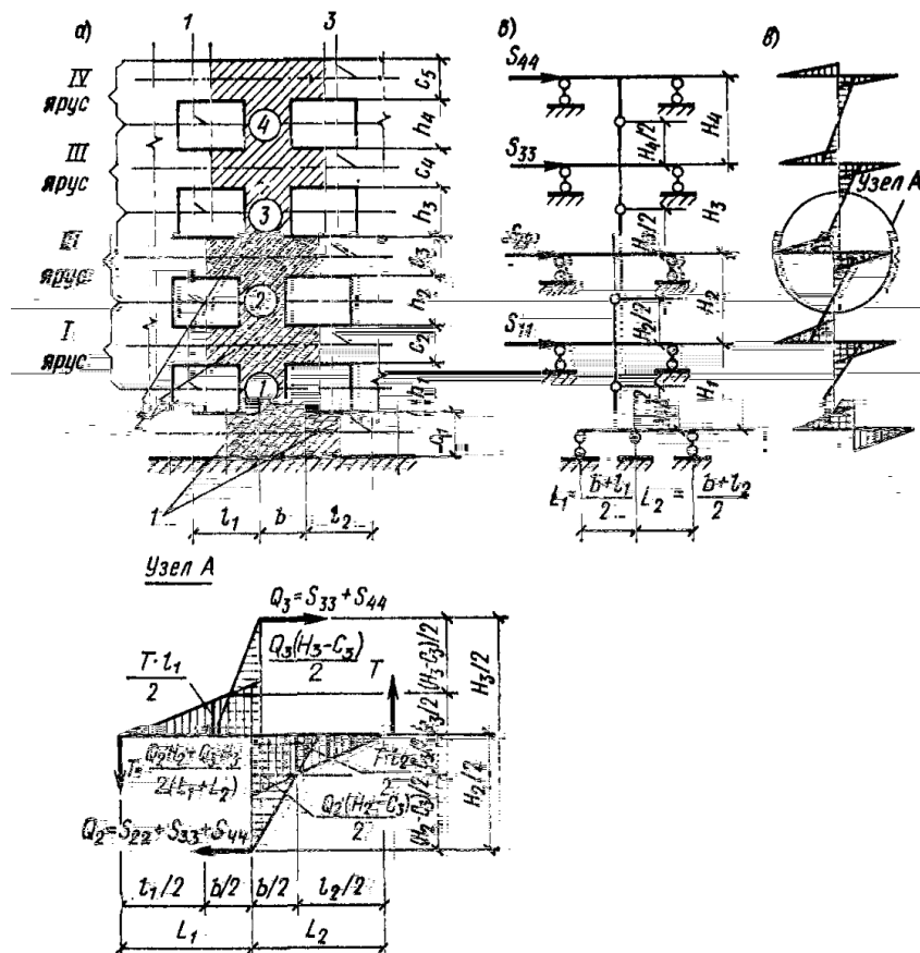
a - элемент фасада стены; b - расчетная схема; c - эпюра M ; d - оси проемов; e - простенки; f - оси горизонтальных поясов
