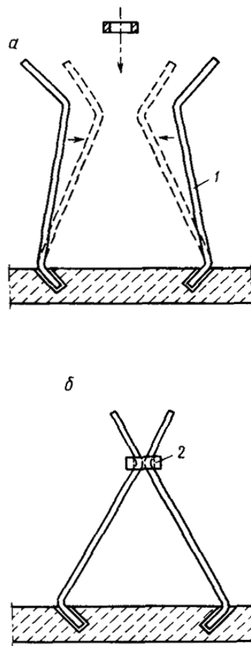
Рис. 14. Установка разъемной закрепы
