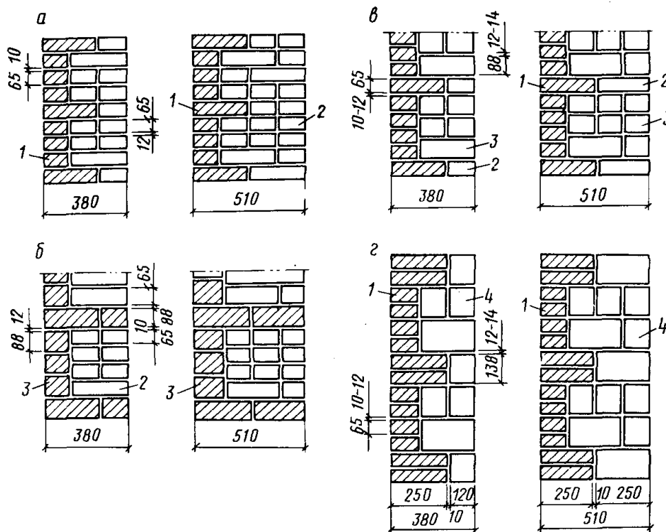
Рис. 1. Облицовка лицевым кирпичом стен
