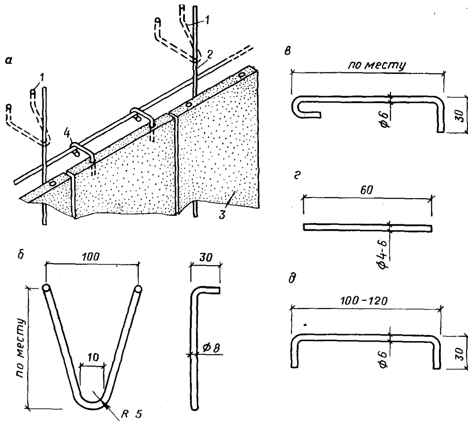
Рис. 5. Крепление облицовочных плит при ведении работ по готовой стене
