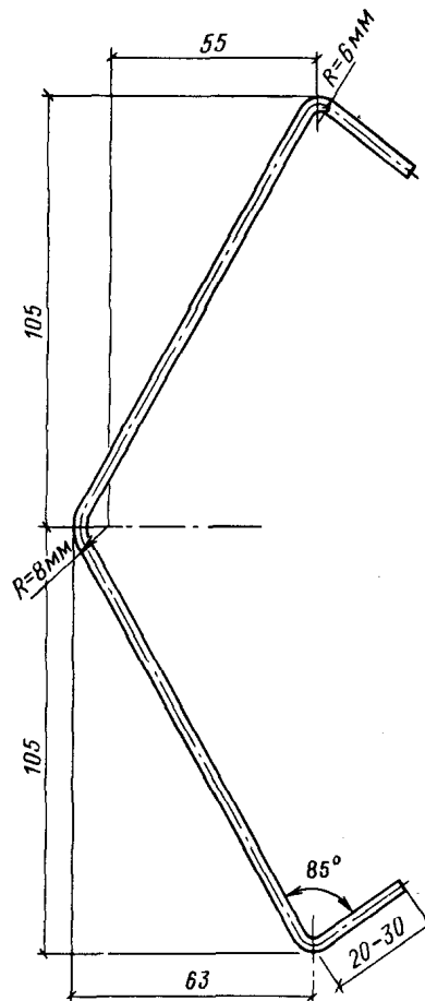
Рис. 13. Пружинная закрепа
