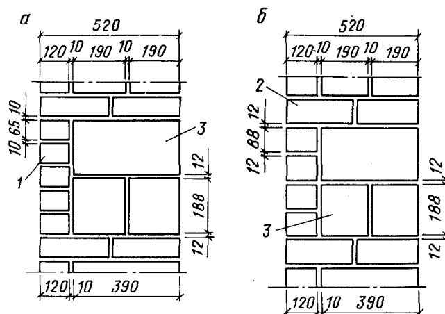
Рис. 4. Облицовка лицевым кирпичом стен из бетонных камней
