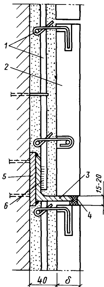
Рис. 6. Вариант устройства компенсационного шва
