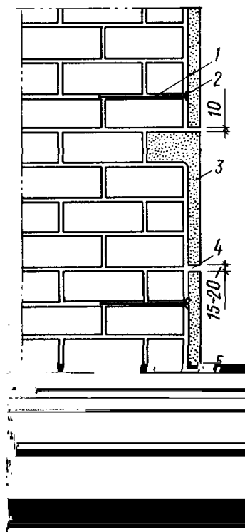
Рис. 12. Кладка из кирпича или камней с облицовкой фасадными бетонными плитами
