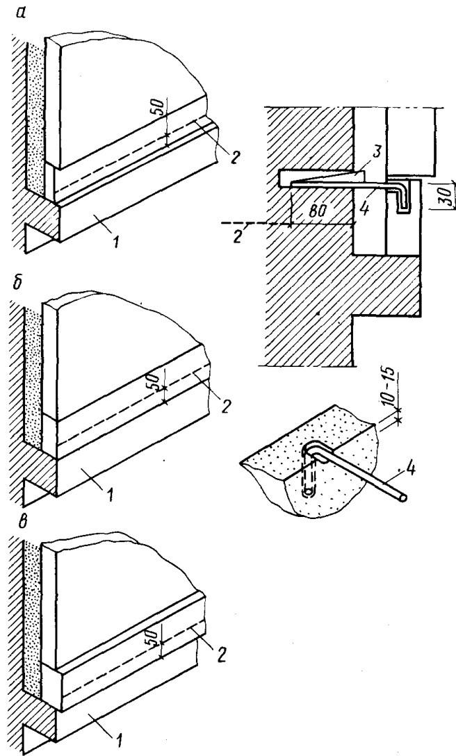
Рис. 7. Облицовка цоколя здания плитами
