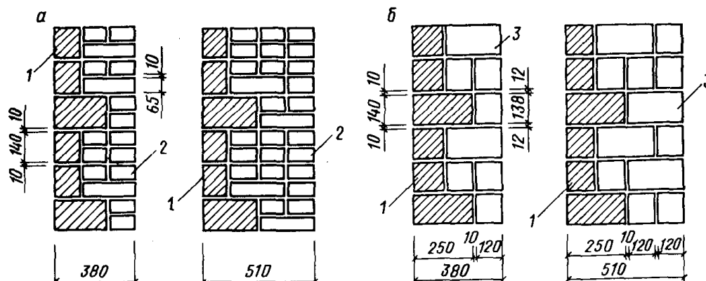
Рис. 2. Облицовка лицевыми керамическими или силикатными камнями стен
