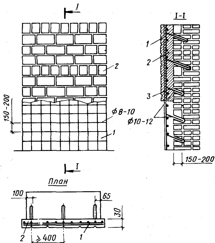
Рис. 17. Пример усиления простенка путем замены разрушенной облицовки железобетонной стенкой
