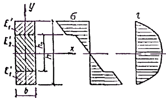
Рис 4 Эпюры нормальных и касательных напряжений неоднородного прямоугольного сечения
