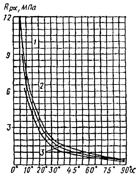
Рис График зависимости расчетных сопротивлений растяжению МПа клееной древесины сосны и ели от угла наклона к волокнам для I и II сортов
