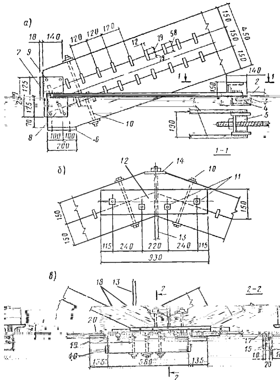
Рис Узлы металлодеревянной треугольной фермы
