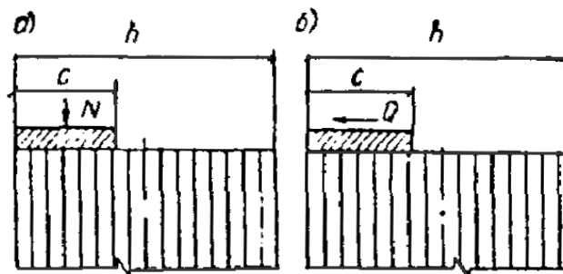
Рис Схема загрузки торца деревянного элемента местной нагрузкой ) вдоль волокон; ) поперек волокон
