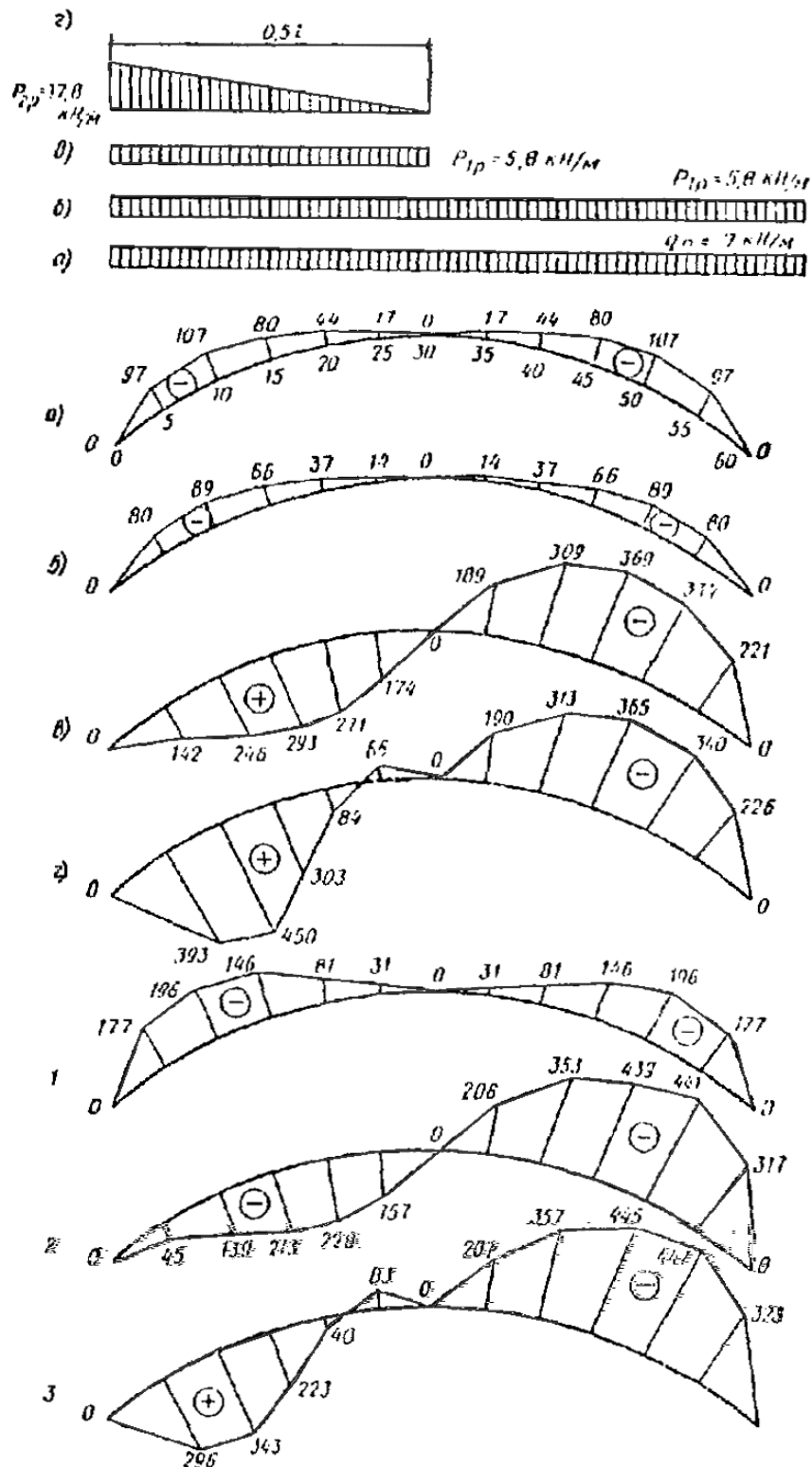
Рис Эпюры изгибающих моментов в арке от расчетных нагрузок и от их сочетания
