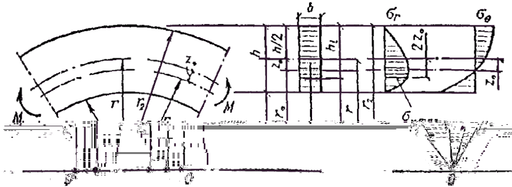
Рис Геометрические характеристики и эпюры радиальных и тангенциальных нормальных напряжений гнутоклееного элемента
