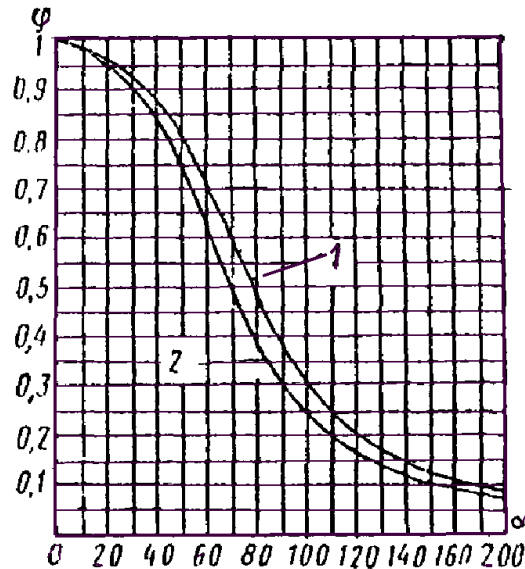
Рис График определения коэффициента продольного изгиба \varphi по формулам и СНиП
