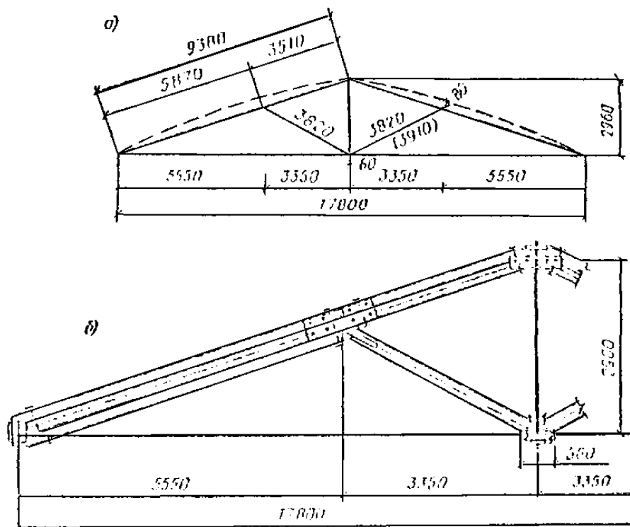
Рис Металлодеревянная треугольная ферма с верхним поясом составного сечения из брусьев на пластинчатых нагелях
