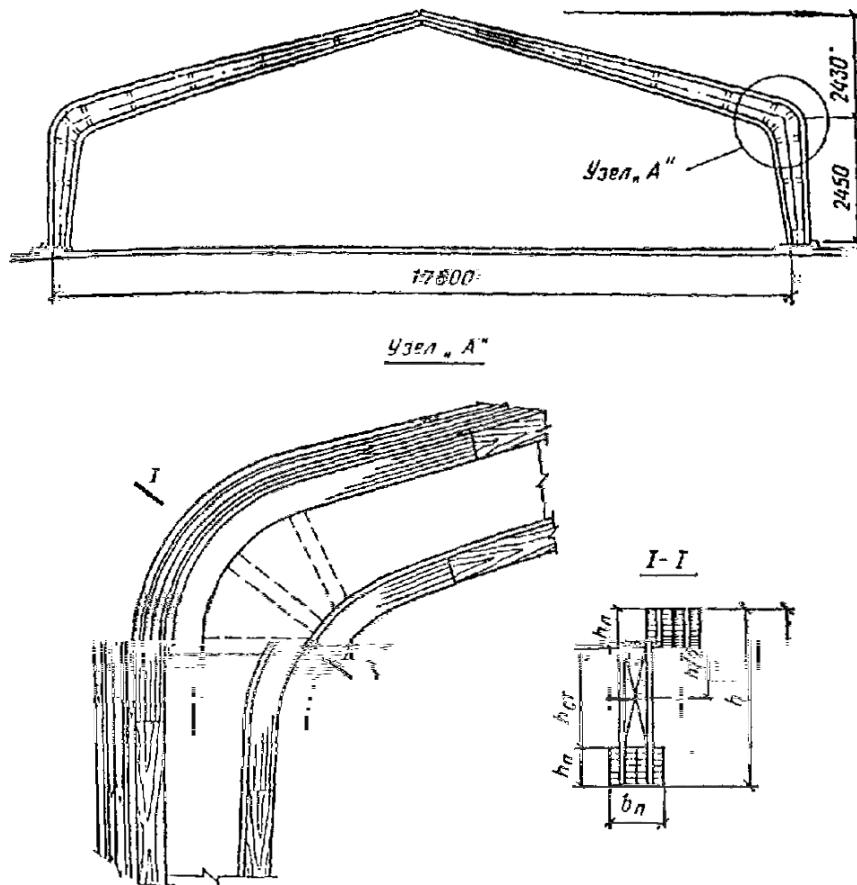
Рис Клефанерная трехшарнирная рама с гнотоклееными вставками в карнизных узлах
