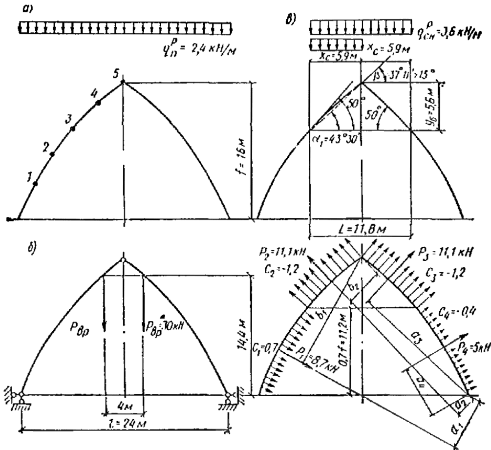
Рис Схема нагрузок действующих на арку
