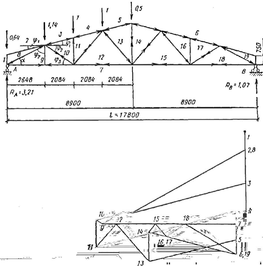
Рис Расчетная схема нагружения фермы и диаграмма усилий в ее элементах
