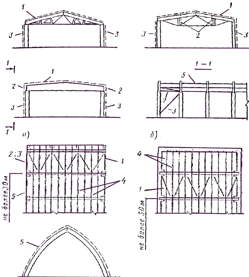
Рис Схемы пространственного крепления плоских деревянных конструкций в зданиях и сооружениях каркасного типа а и без каркаса б
