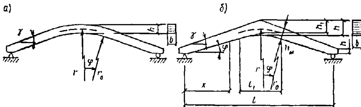
Рис Гнутоклееные балки
