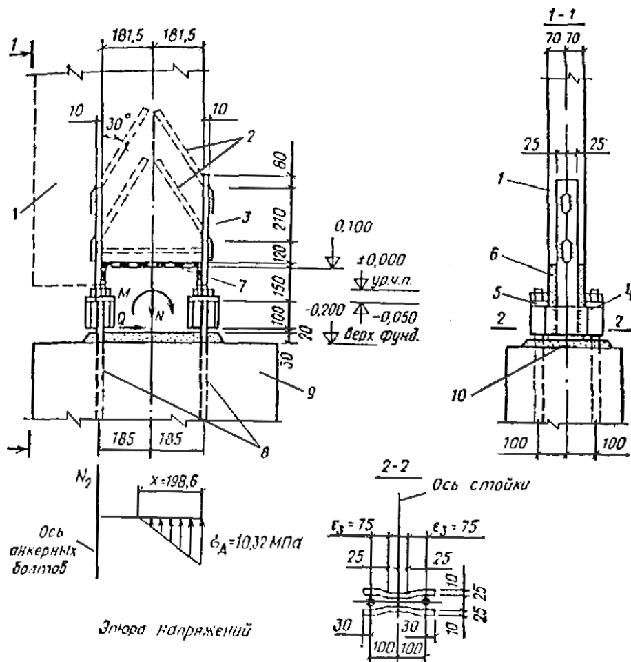
Рис Опорный узел рамы
