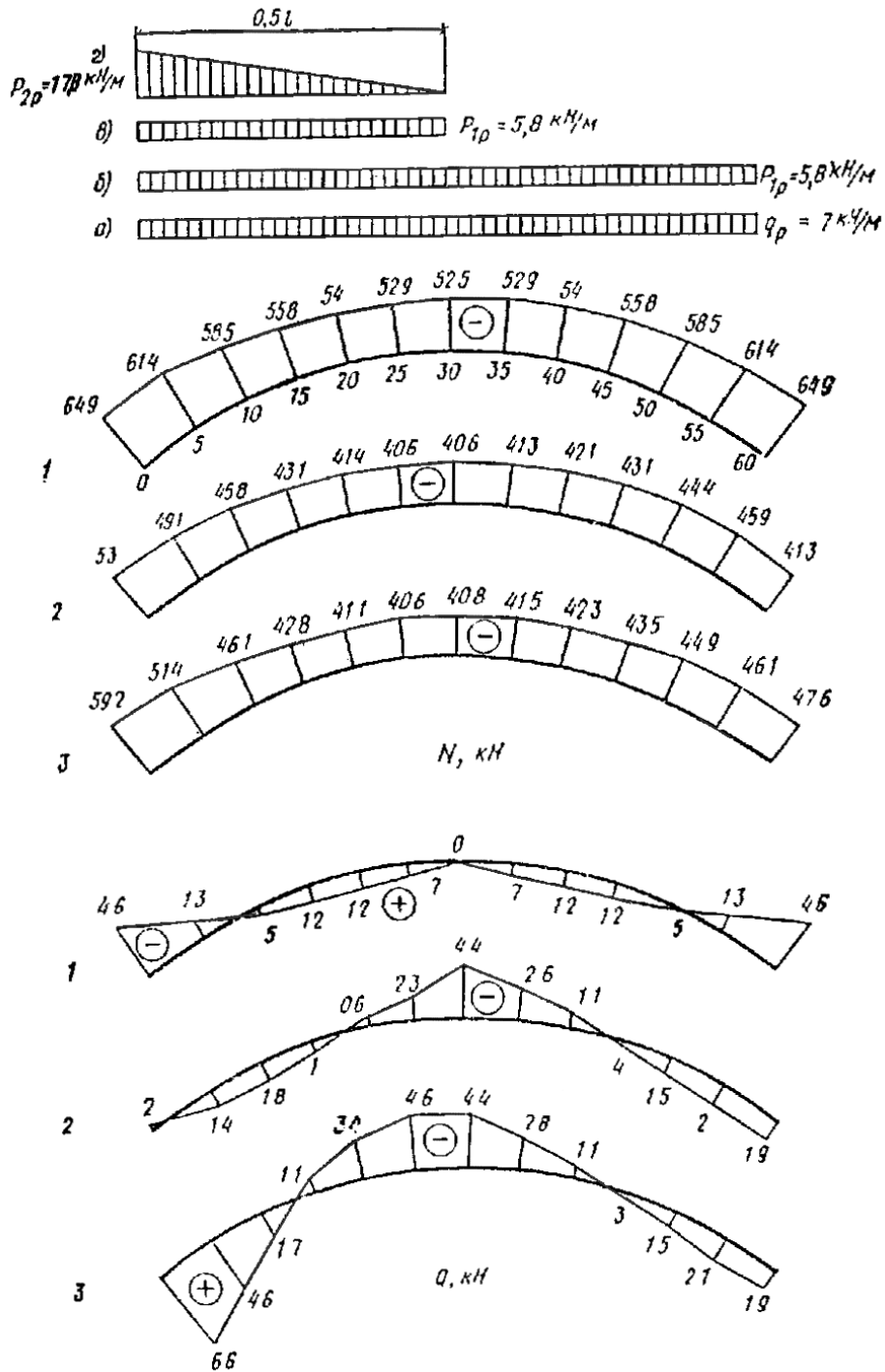
Рис Эпюры нормальных N и поперечных Q сил в арке от сочетания расчетных нагрузок
