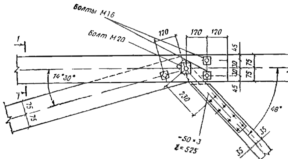
Рис Узел Б брусчатой фермы
