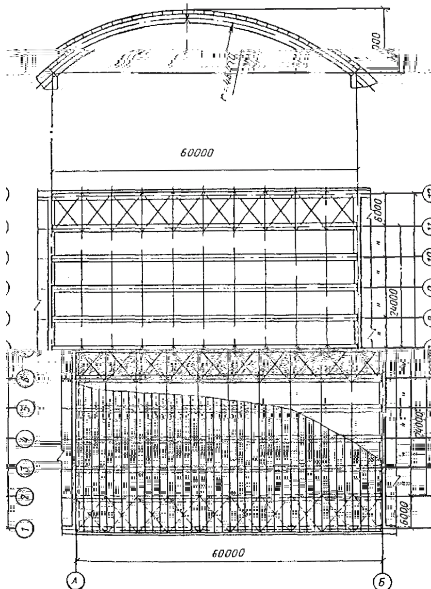
Рис Поперечный разрез и план арочного покрытия
