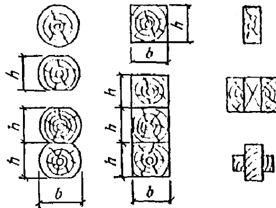
Рис Примеры компоновки поперечного сечения элементов из цельной древесины
