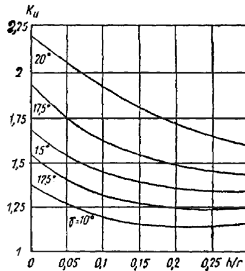
Рис График для определения коэффициента K_u при расчете гнутоклееных балок переменной высоты
