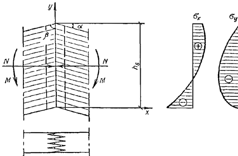
Рис Соединение клееных элементов на зубчатый шип под углом по всему сечению
