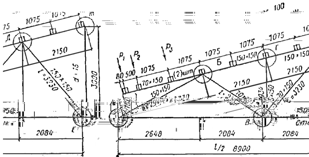
Рис Геометрическая схема фермы
