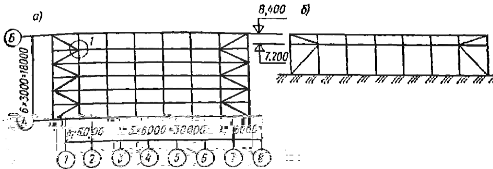
Рис Схема продольных и поперечных связей жесткости
