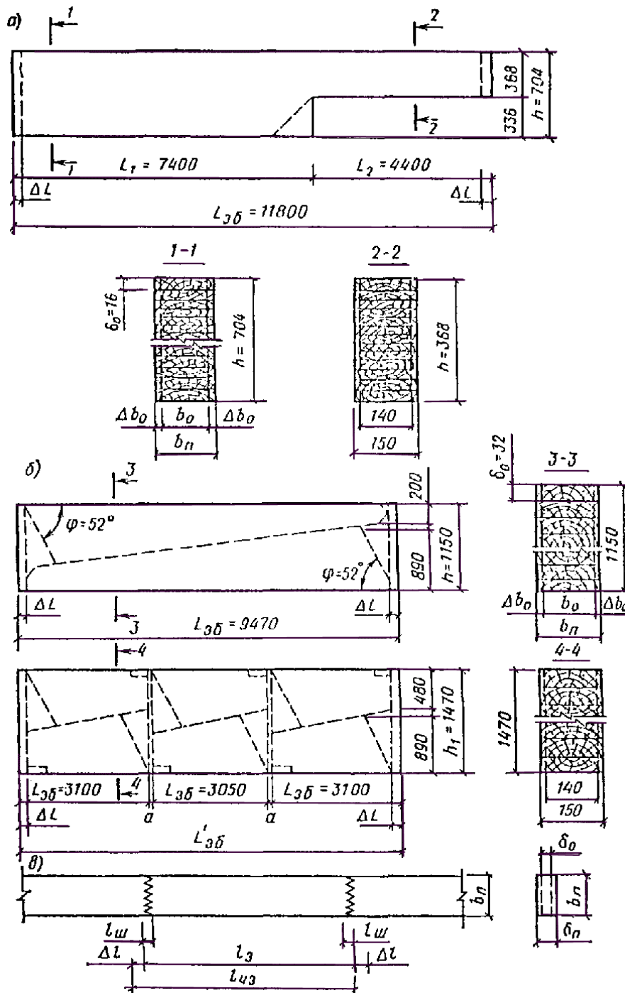
Рис Заготовочные блоки
