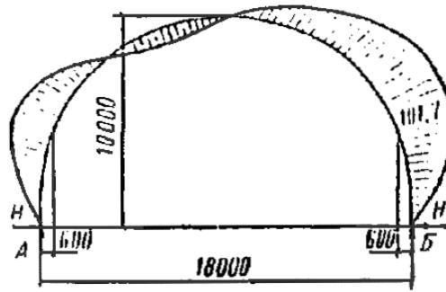
Рис Эпюра расчетных изгибающих моментов
