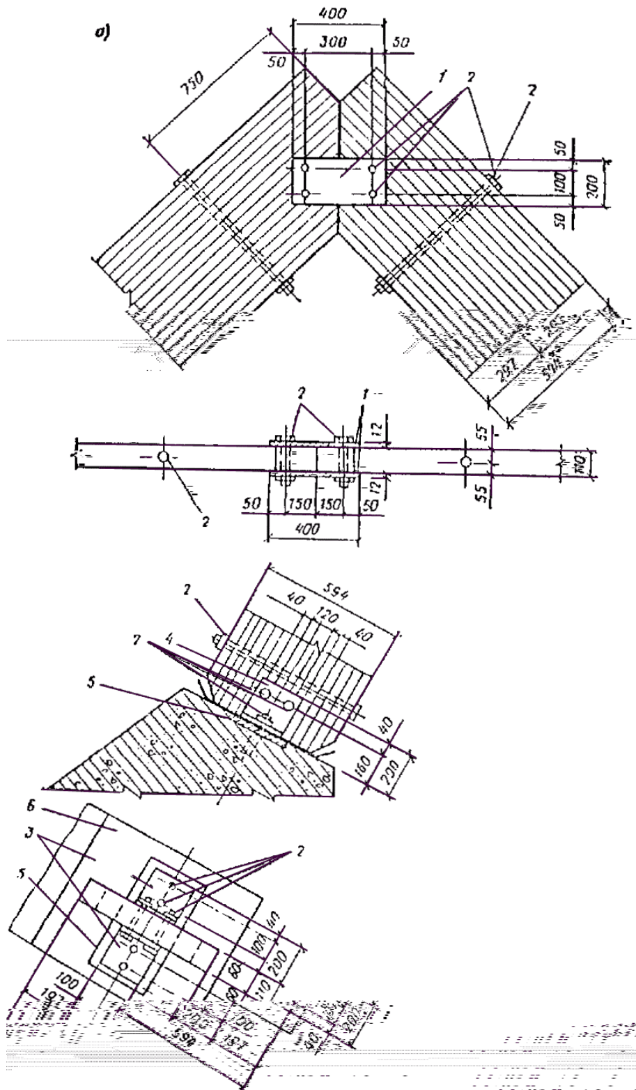
Рис Коньковый а и опорный б узлы стрельчатой арки
