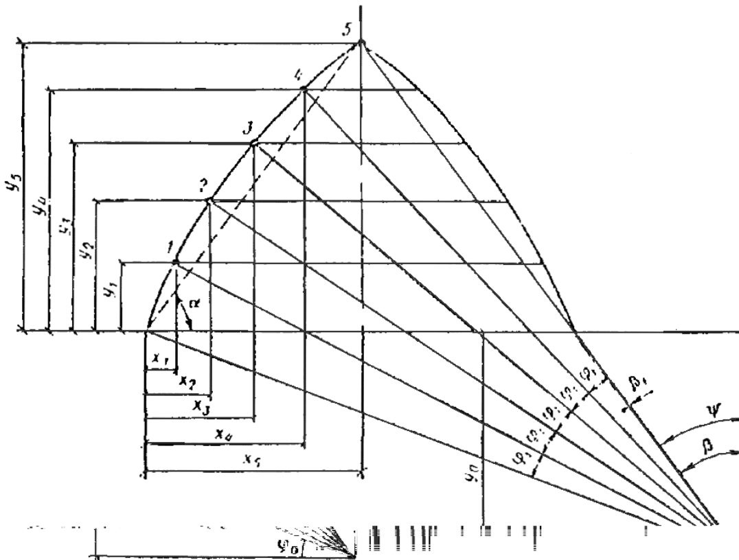
Рис Построение геометрической оси арки
