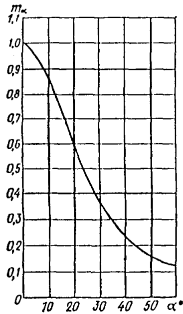
Рис График зависимости коэффициента m_\alpha от угла наклона волокон к определению расчетного сопротивления изгиба R_{II} при проверке прочности внешне растянутой кромки узлового соединения на зубчатый шип
