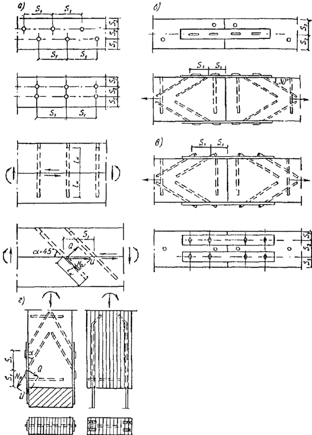
Рис Соединения на клеенных в древесину стержнях из арматурной стали
