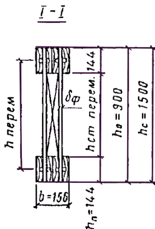
Рис Двускатная клефанерная балка покрытия
