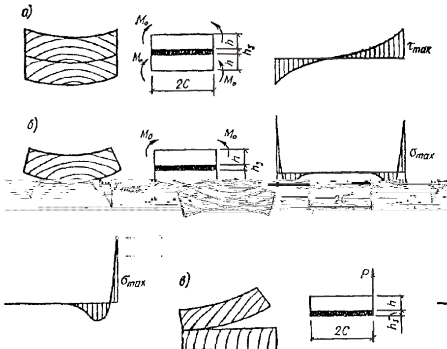
Рис Характер распределения собственных внутренних нормальных и касательных напряжений поперек волокон возникающих при высыхании клееной древесины в случае трех типичных сочетаний досок с различным расположением годовых слоев в сечении
