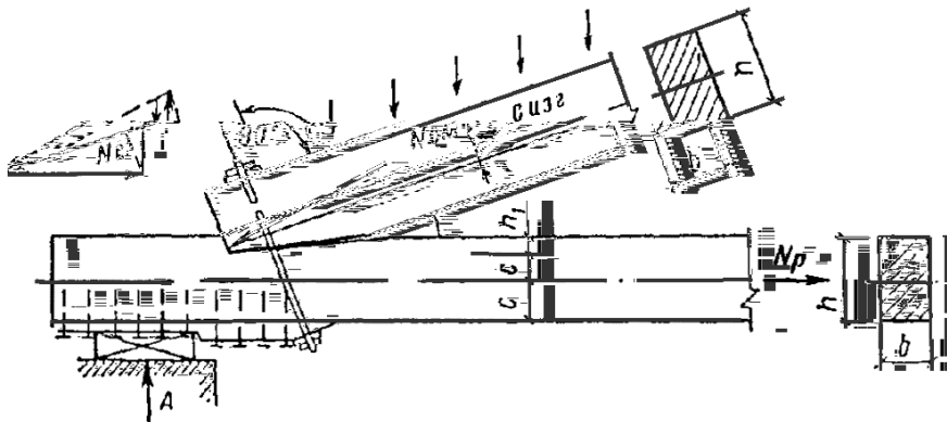
Рис Лобовая врубка с одним зубом при внеузловой нагрузке
