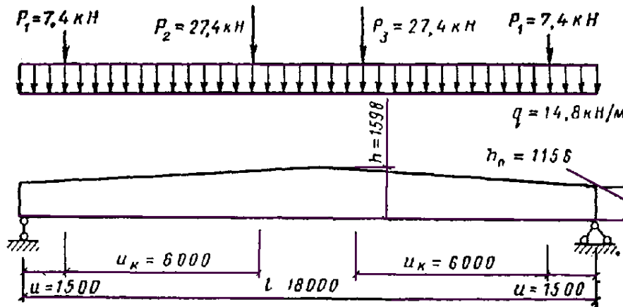
Рис Расчетная схема дощатоклеенной балки покрытия с подвесным оборудованием
