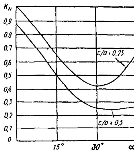
Рис График зависимости коэффициента K_N от угла наклона волокон \alpha и параметра c/a
