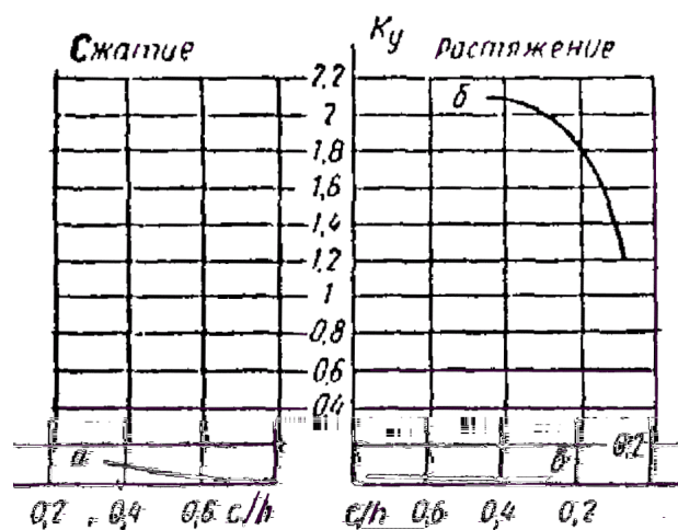
Рис График для определения коэффициента концентрации напряжений поперек волокон K_y
