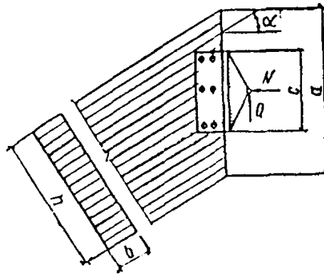
Рис Конструктивная схема ключевого шарнира арки к определению коэффициента K_N
