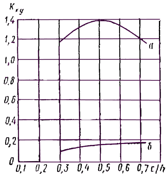
Рис График для определения коэффициента концентрации касательных напряжений K_{xy}
