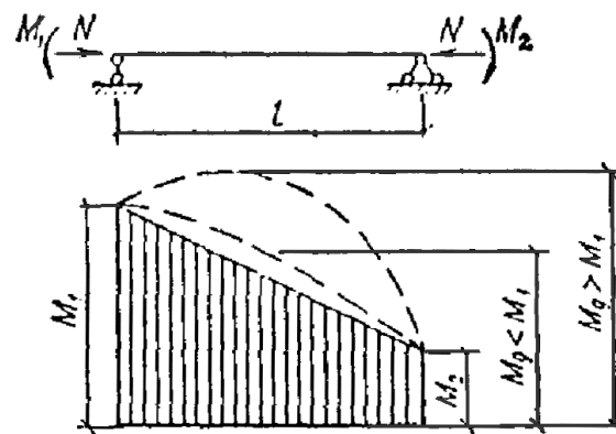
Рис Эпюры моментов сжато изгибаемого элемента из расчета по деформированной и недеформированной схемам
