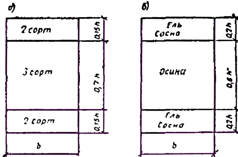
Рис Примеры компоновки сечения дощатых клееных балок
