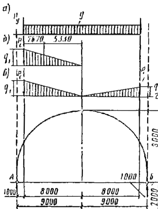
Рис Расчетная схема рамы с нагрузками a постоянная нагрузка от собственного веса б в снеговая нагрузка
