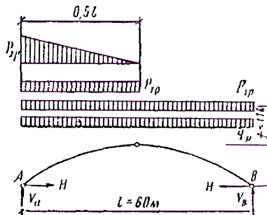
Рис Схема нагрузок от собственного веса и снега действующих на арку
