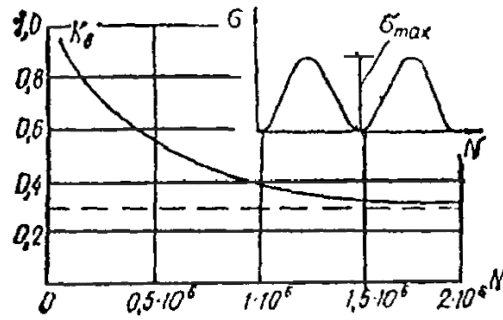
Рис График зависимости коэффициента выносливости древесины от числа циклов N при изгибе
