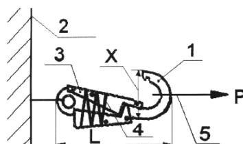
Рисунок 8а - Схема испытания карабина статической нагрузкой
