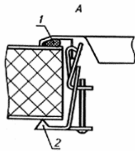
1 - прокладка; 2 - зажим
